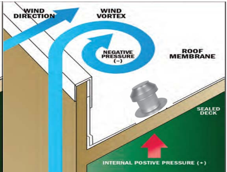
ERS VORTEX Roofing System
